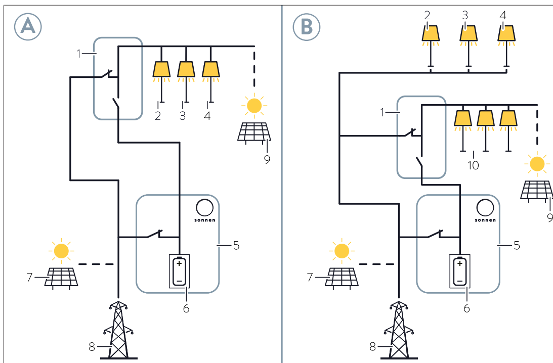
Abb. 7: Normalbetrieb - kein Netzausfall (A: Anschlussvariante 1; B: Anschlussvariante 2)
